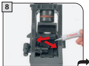
8 Solo con il grasso fornito in dotazione, lubrificare le guide del gruppo.
